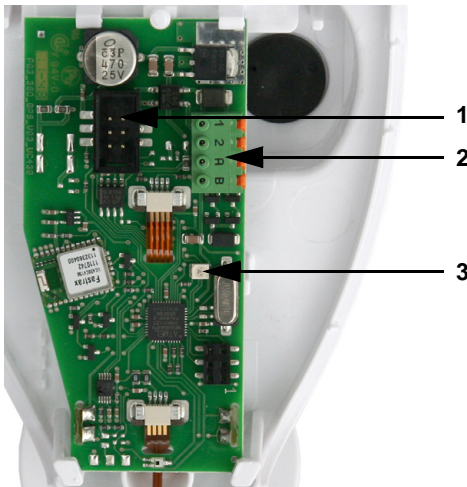
Abb. 12: Übersicht Platine
