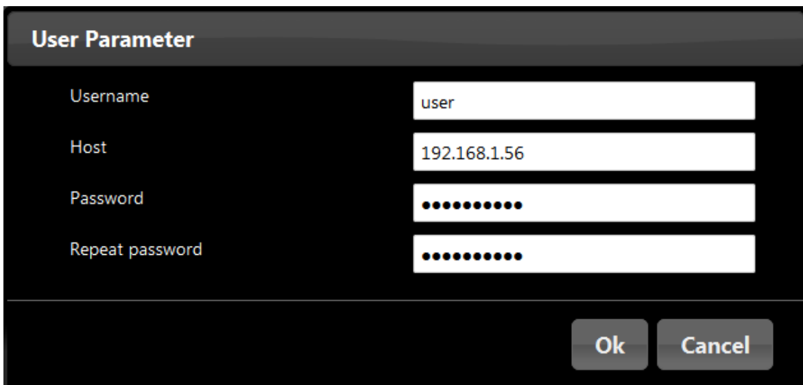
Figure 24: User Parameter
